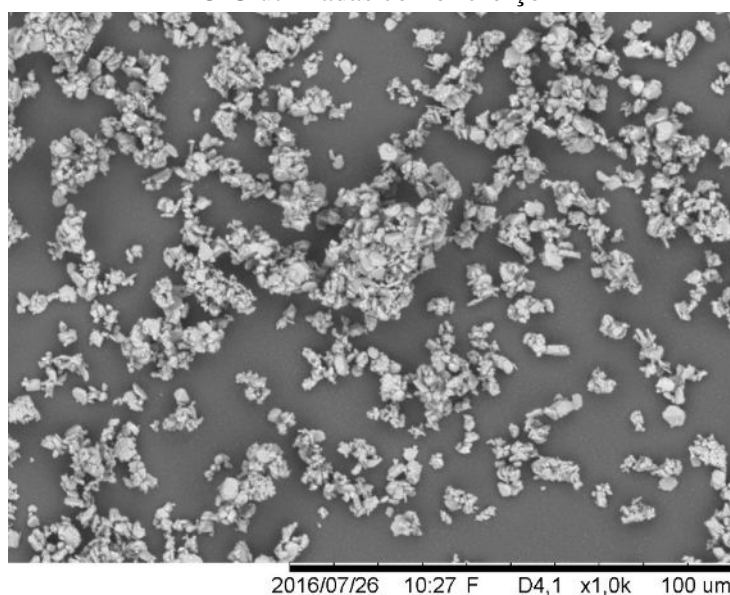
Figura 3 - Micrografia das partículas de alumina calcinada APC-G utilizadas como reforço
