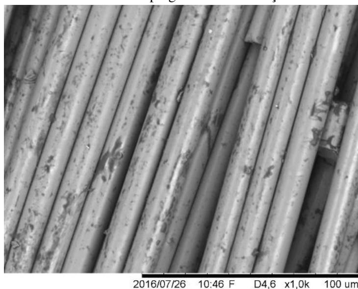
Figura 2 - Micrografia da superfície das fibras de vidro cortadas empregadas como reforço
